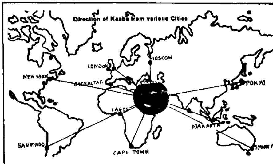
DE GEBEDSRICHTING VAN KAABA VANUIT VERSCHILLENDE STEDEN
